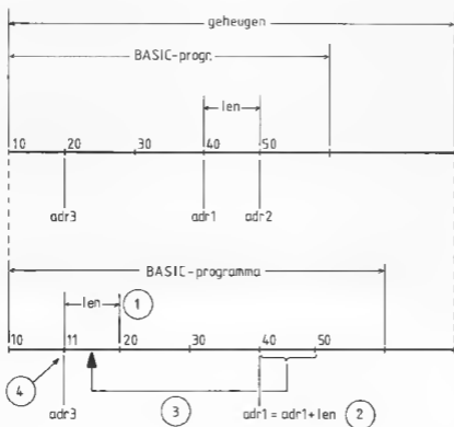
Atb. 9-1 Geheugenindeling bij kopiëren
